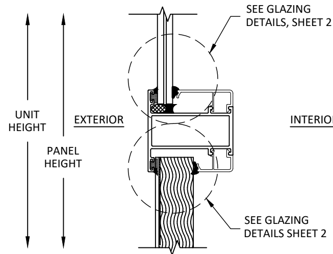
H 11 VERTICAL SECTION ALS MIDRAIL - INFILL OVER INFILL NON - REINFORCED
