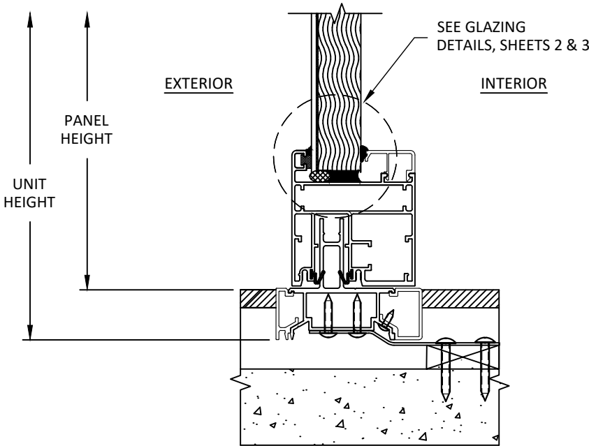
CC 13 VERTICAL SECTION ALS SILL H TRACK
