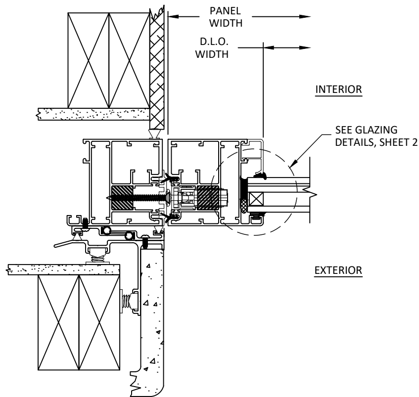
L 14 HORIZONTAL SECTION ALS 1-TRACK POCKET JAMB
