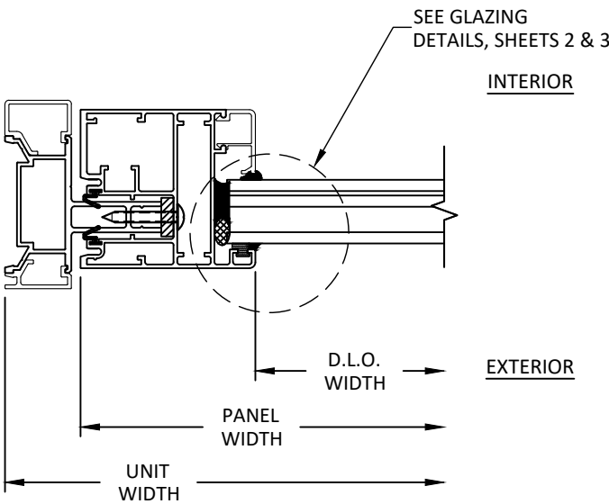
AA 13 HORIZONTAL SECTION ALS JAMB H-TRACK
