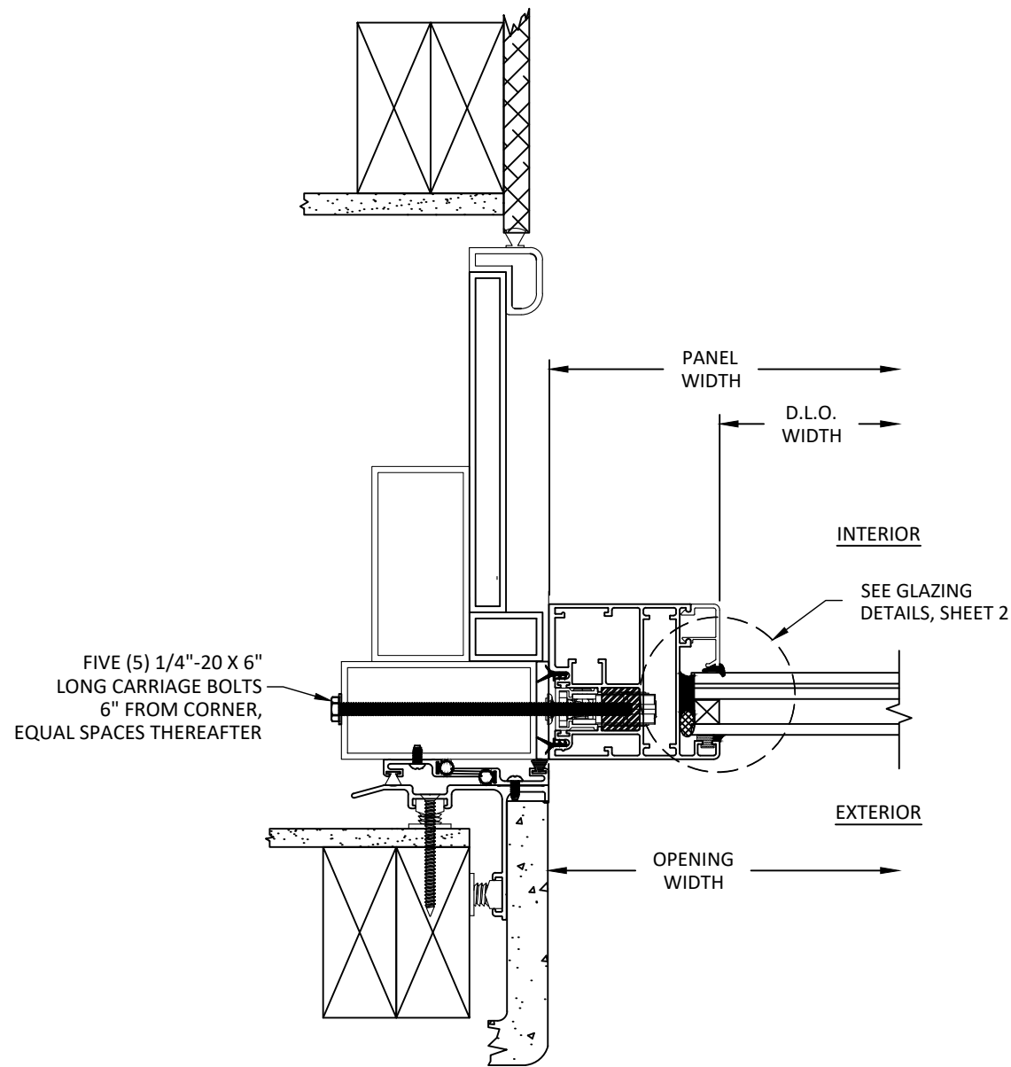
J 14 HORIZONTAL SECTION ALS 3-TRACK POCKET JAMB
