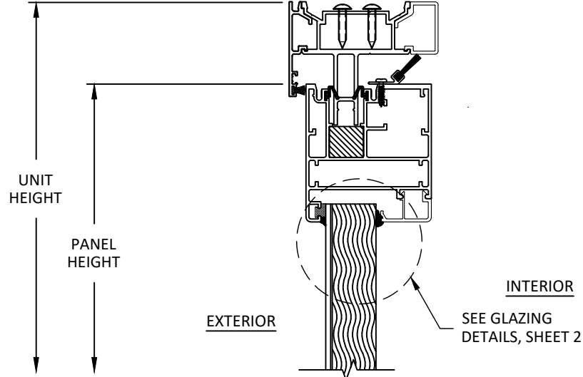
AA 11 VERTICAL SECTION ALS HEAD H TRACK
